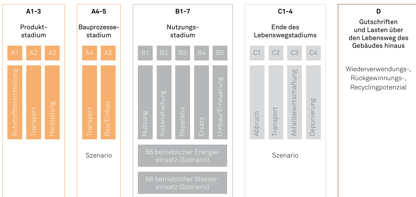
Abbildung 3: Einteilung des Gebäudelebenszyklus nach DIN EN 15804 [12] (Quelle: Fraunhofer IBP [6])
